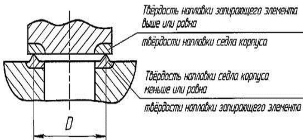
Рисунок Е.1 Плоское уплотнение в затворе
